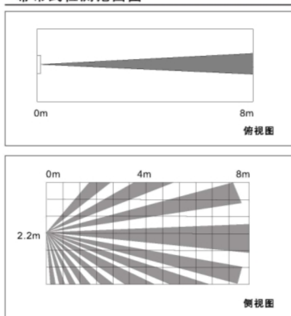
幕帘式检测范围图
